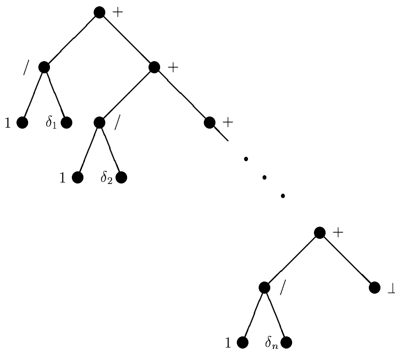
Rysunek 4: Drzewo etykietowane \sigma_n , n -ta aproksymacja drzewa \sigma .
